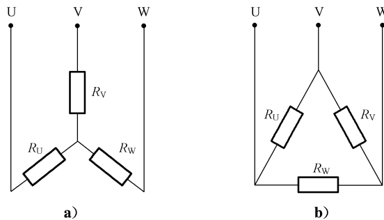
图 1 绕组形式
