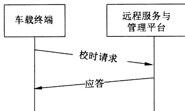
图 B.6 终端校时流程图
