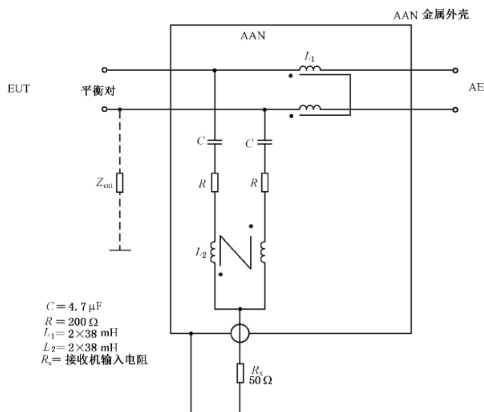
图 B.1 ISN 对称通信线的示例
