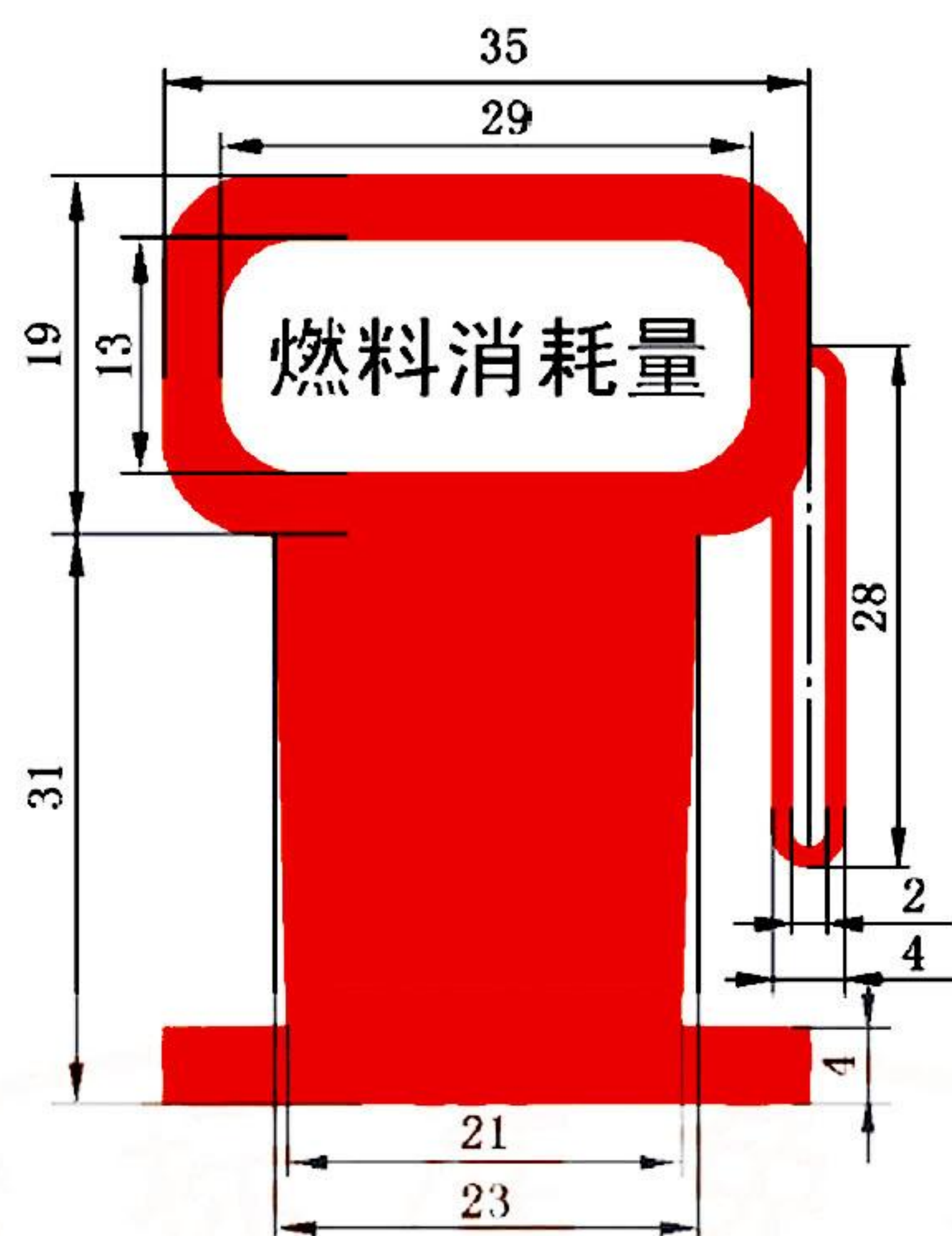
图 A.3 加油机图案及规格要求
